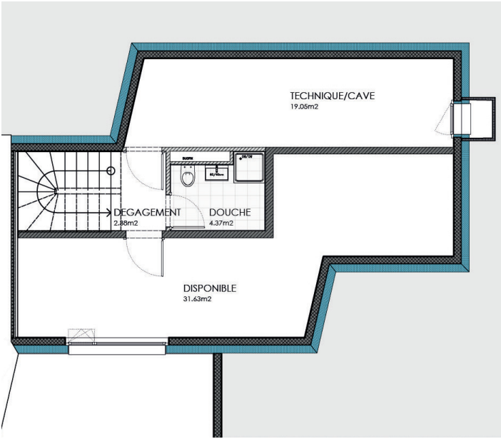
Sous-sol
