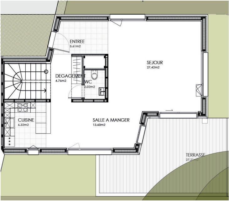
Rez-de-chaussée
